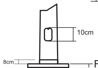
Detalle base:
